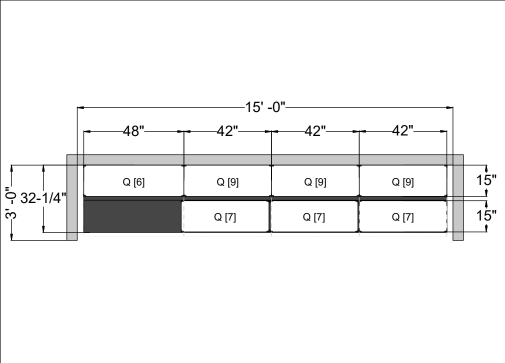
Elevation B
