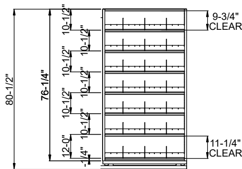
Elevation B
