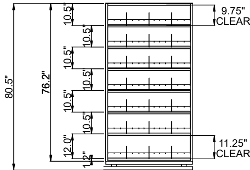
Elevation B
