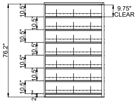
Elevation A
